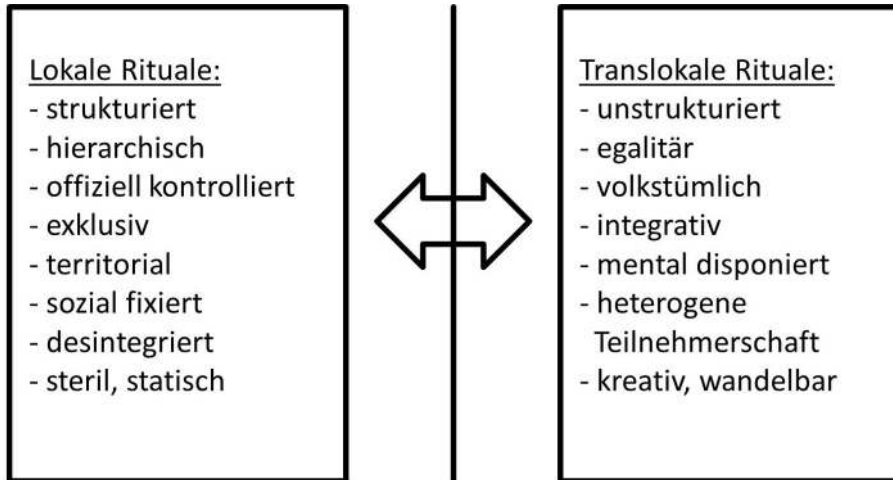
Abb. 1 Dichotomische Bestimmung von lokalem und translokalem Ritual.
